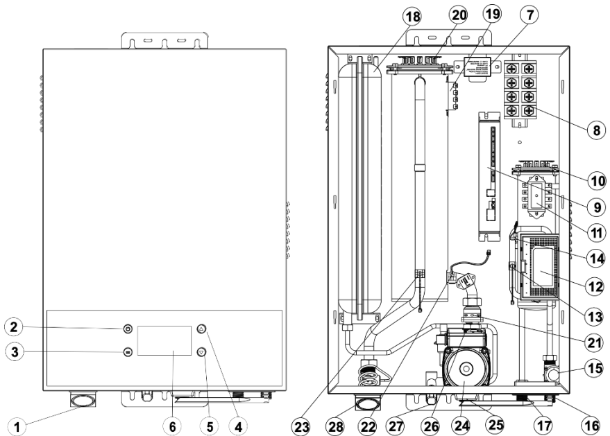
Рис. 1. Конструкция изделия
