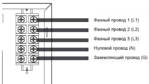
Рис.12. Подключение прибора
