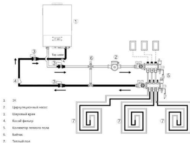
Рис. 6. Схема подключения «тёплый пол + ЭК»
