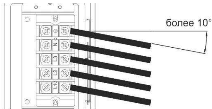
Рис. 10. Расположение сетевого кабеля
